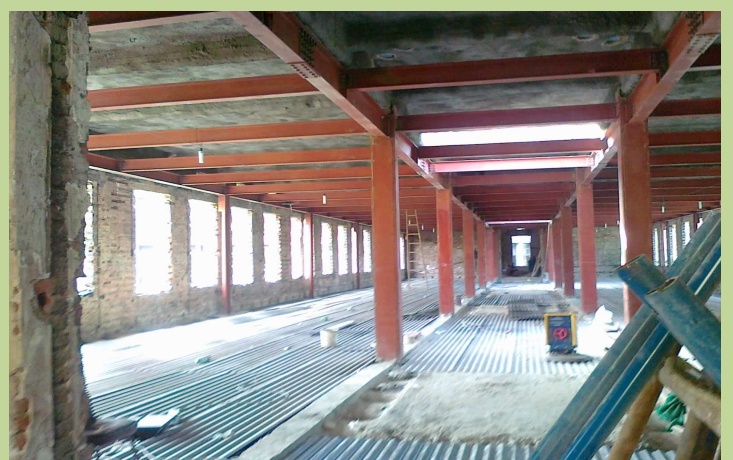
أعمال التدعيم المعدنى للدور الثاني فوق الأرضى بمبنى الإدارة.
