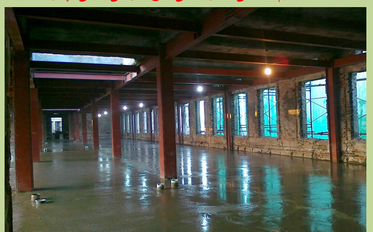
أعمال تدعيم الأرضية بطبقة خرسانية خفيفة.
